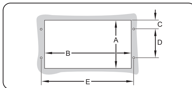
Dimensiones del patrón de la serie RMB2
