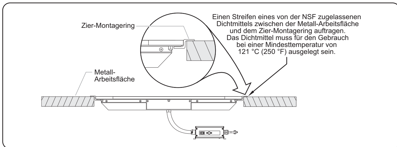
Arbeitsflächenmontage – HBGB
