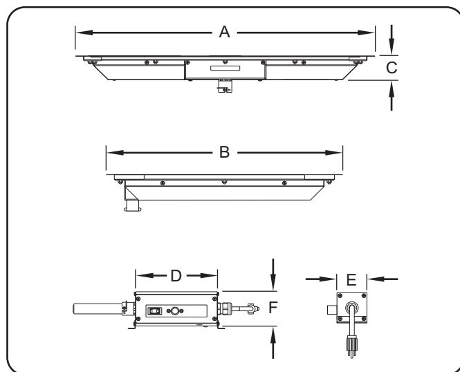
HBGB Dimensions
