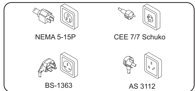
Steckerkonfigurationen
