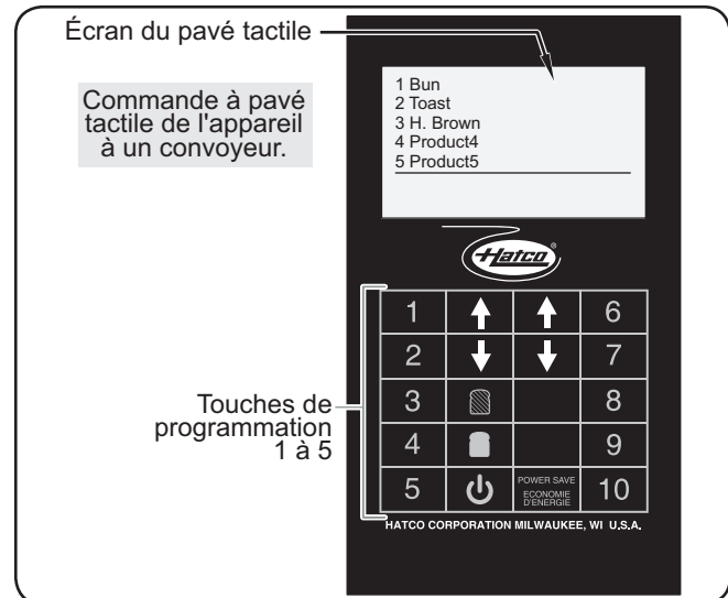
Commande à pavé tactile et écran (illustration de l'ITQ-875-1C et l'ITQ-1000-1C)
