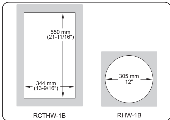
Abmessungen der Öffnung in der Tischfläche
