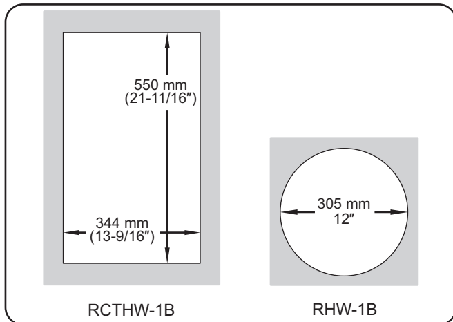
Uitsnijafmetingen aanrecht
