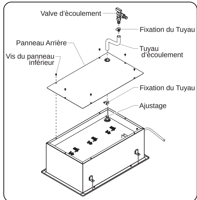
Installation de l'ensemble de vidange (modèles rectangulaires intégré seulement)
