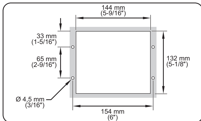
Dimensiones del Hueco para el Panel de Control Externo
