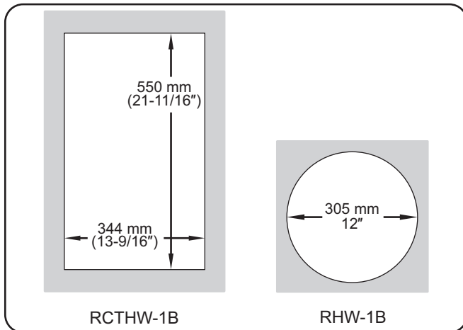
Dimensioni dell'apertura nel piano di lavoro
