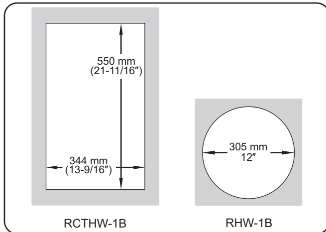
Dimensiones del Hueco del Mostrador
