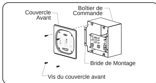
Installation du Boîtier de Commande Monté à Distance
