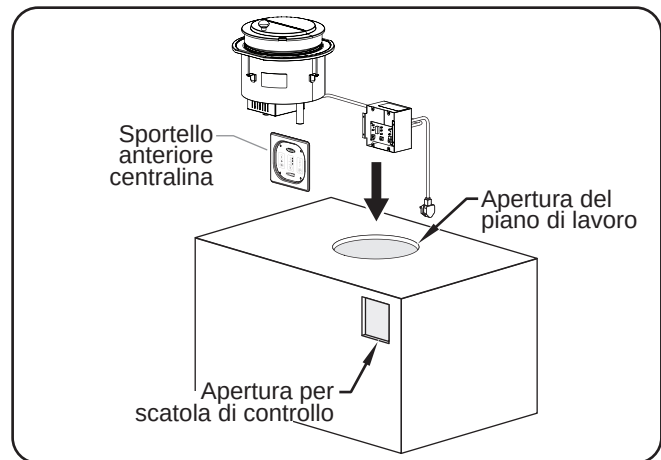
Installazione dell'unità
