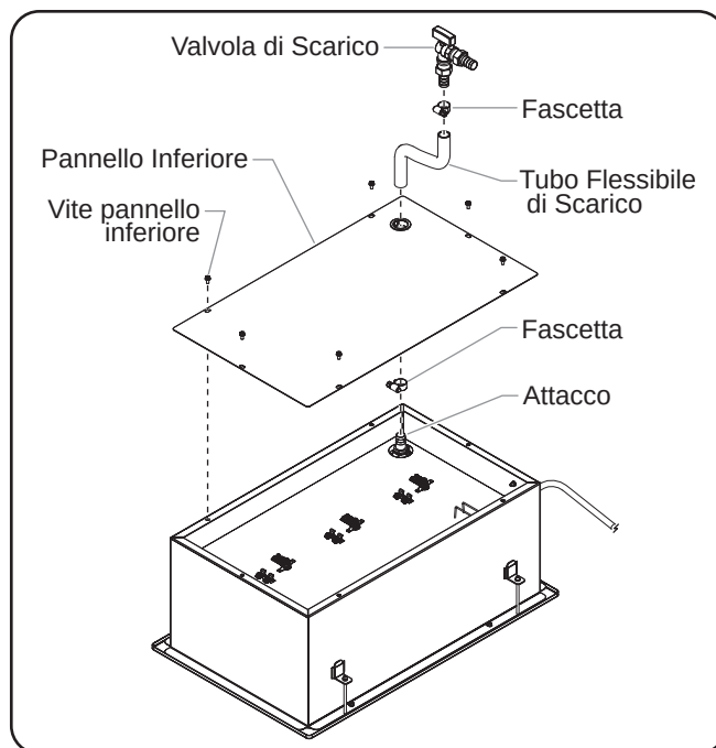
Installazione del gruppo di scarico (solo modelli incassati rettangolari)
