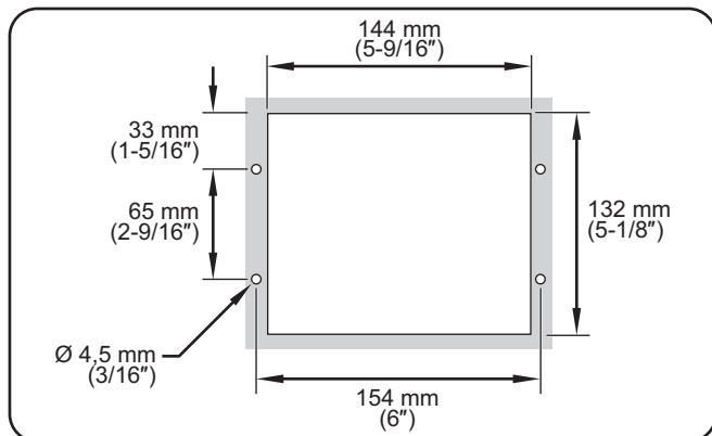
Uitsnijafmetingen bedieningspaneel
