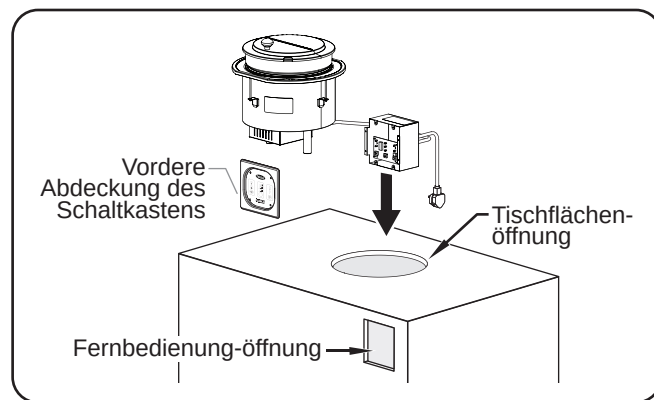
Einbau des Geräts
