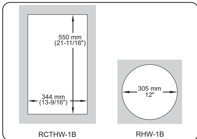
Dimensions des Découpes de Comptoir
