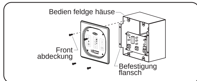
Einbau der Fernbedienung
