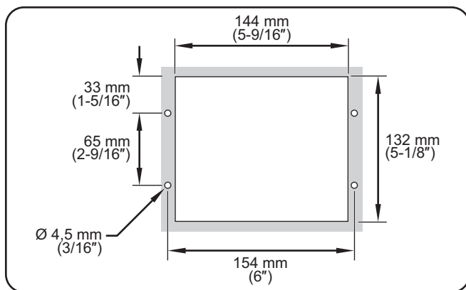
Dimensioni dell'apertura per la scatola di controllo
