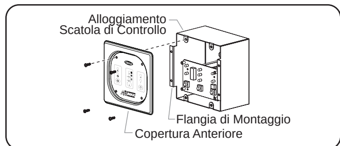
Installazione La Scatola del Comando a Distanza
