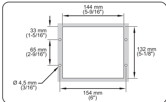
Abmessungen der Öffnungen für die Fernbedienung
